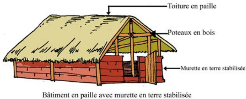
Figure 18. Bâtiment en paille avec murette en terre stabilisée
